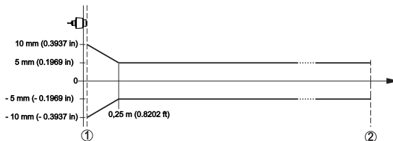
Figure 12.3 Écart de mesure sous conditions de référence 2
